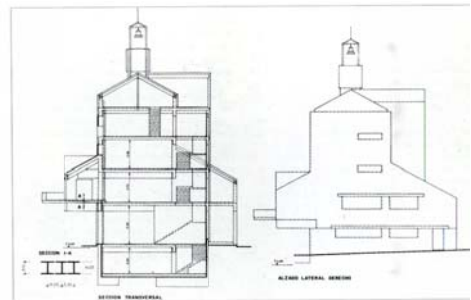
Sección transversal y alzado lateral derecho.
